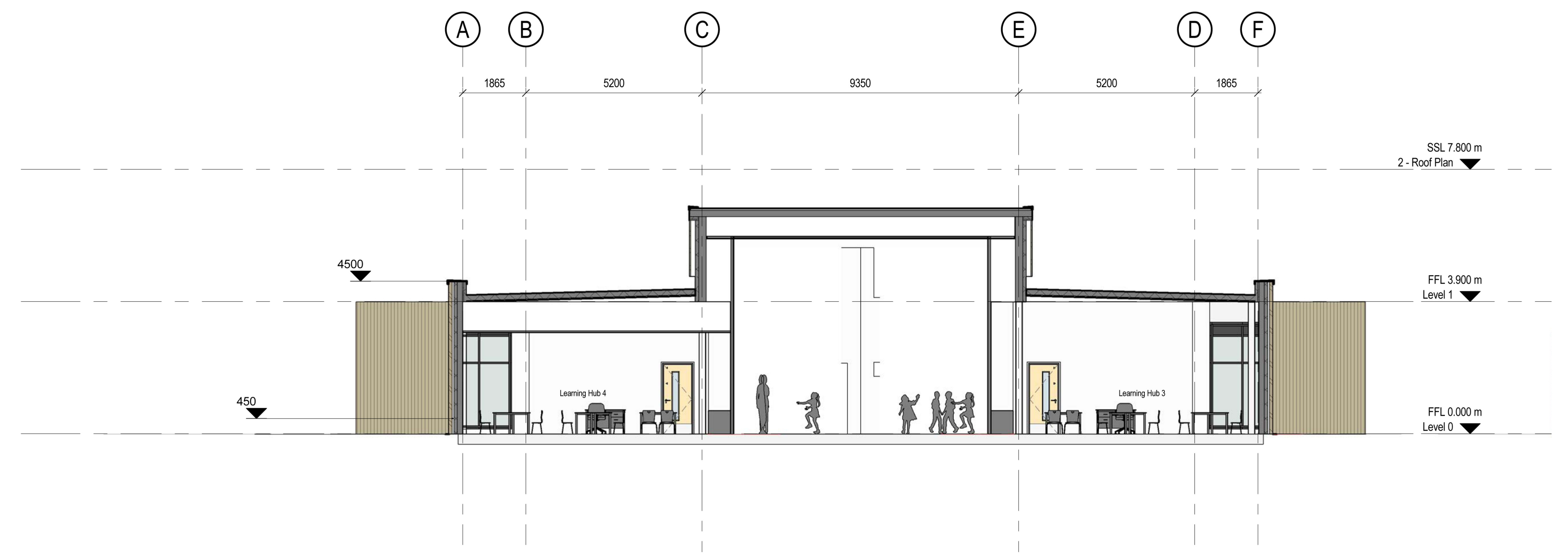
Section A-A 1:100
